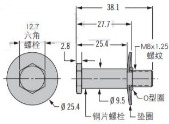
钢片螺栓装置—标准(另外订购)
