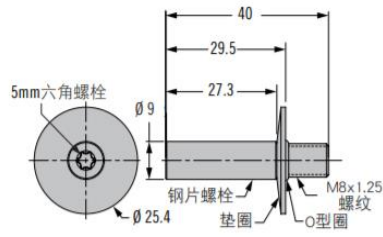
钢片90°安装支架
