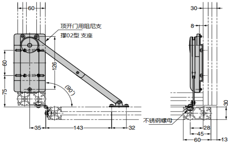
【安装尺寸图】
