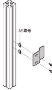
【吸片安装方法】
