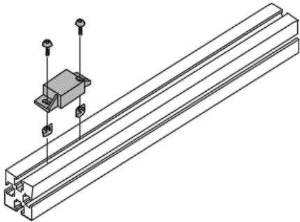
安装方法
