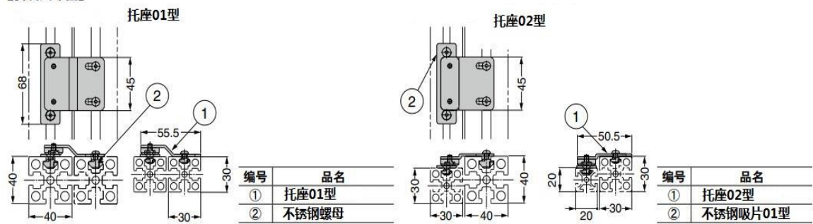
【安装尺寸图】
